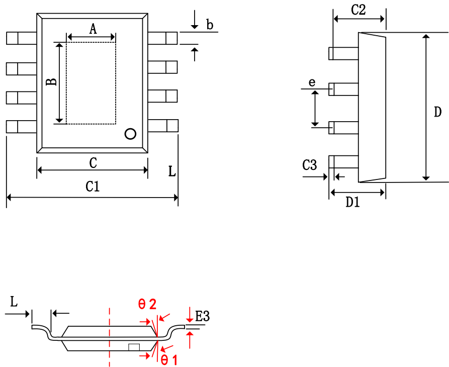
ESOP-8
