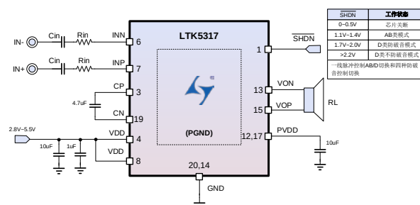
图1. LTK5317应用原理图
