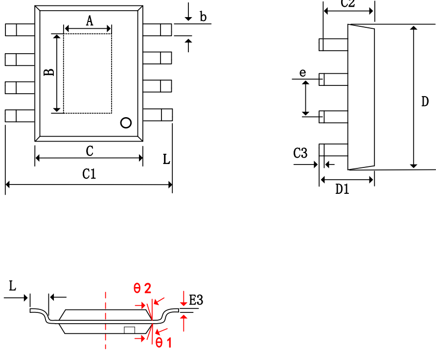
ESOP-8
