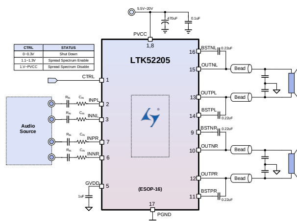
图1. LTK52205 简化应用原理图
