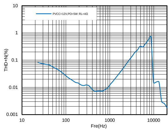
图25. 频率失真曲线
