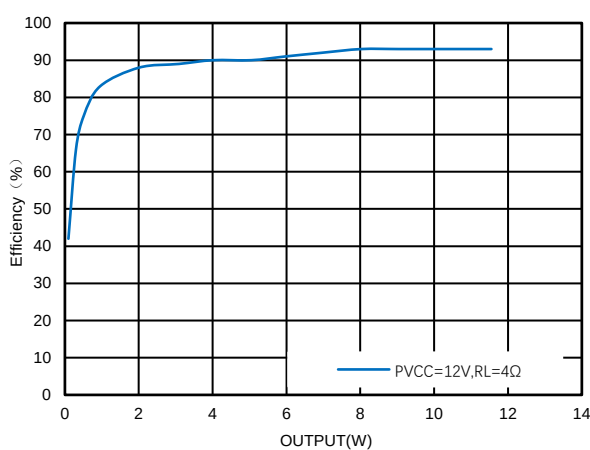
图24. 效率曲线
