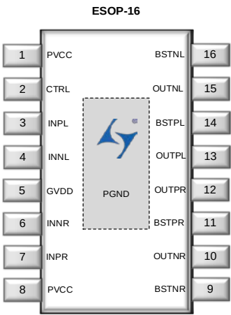
图2. LTK52205 管脚说明
