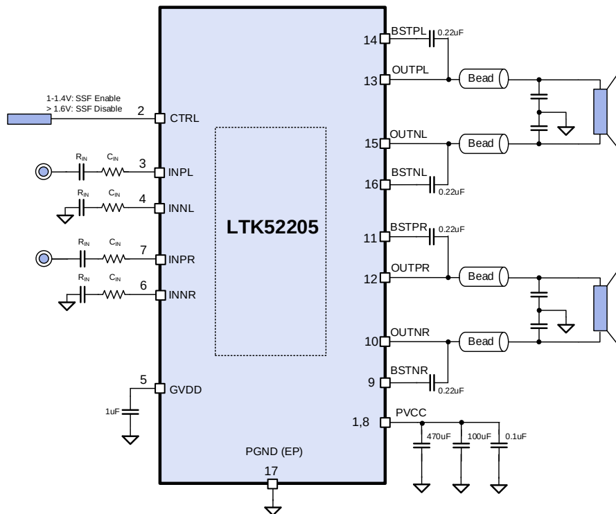
图 5. 单端输入立体声 BTL 输出模式
